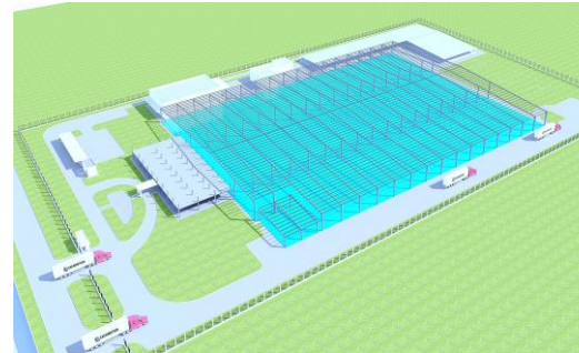
KHUNG KẾT CẤU THÉP/ STEEL STRUCTURE
